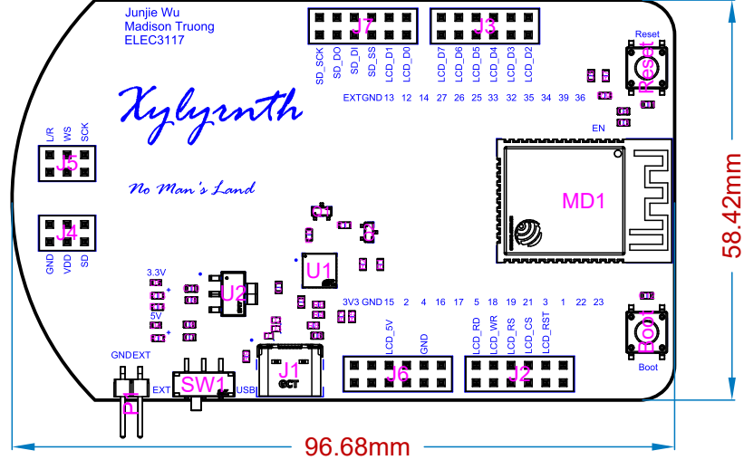
Top side (Scale 1:1)
