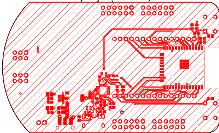
Top Layer (Scale 1:1)
