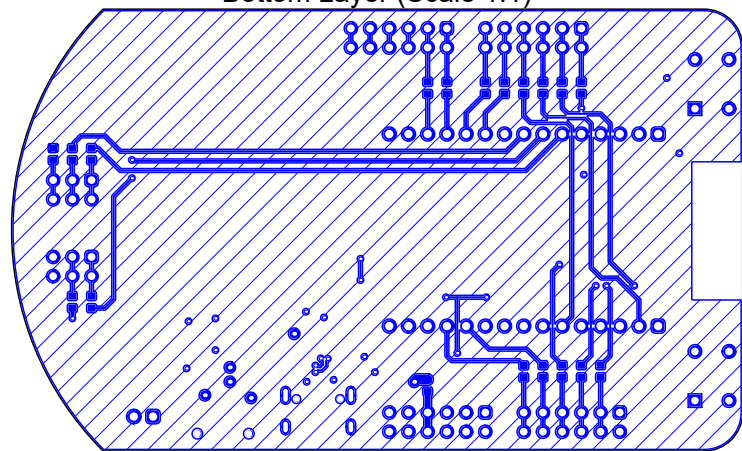
Bottom Layer (Scale 1:1)
